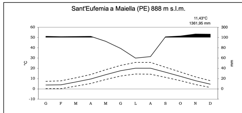
Diagramma ombrotermico dalla stazione di S. Eufemia a Maiella (PE), 1980-2014.
